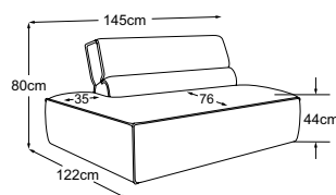
Elemento 2p con terminale sx
