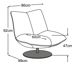
Softie fauteuil (avec pied de plat) N° de commande : D077100
