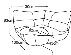
Angle trapézoïdal
