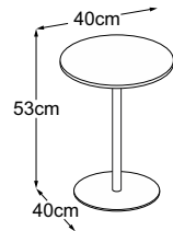
Center Leg 53 (Tischplatte: Struttura Verde) Bestell-Nummer: DCL5SV5
