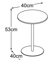
Center Leg 53 (Tischplatte: Vetro Bianco) Bestell-Nummer: DCL5VB5
