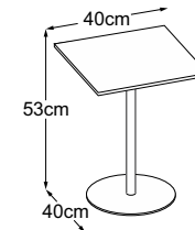
Center Leg 53 (Tischplatte: Struktura Grigio Chiaro) Bestell-Nummer: DCL5SC6
