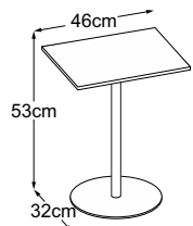
Center Leg 53 (Tischplatte: Struktura Verde) Bestell-Nummer: DCL5SV7
