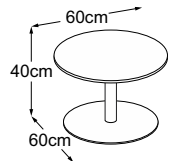
Center Leg 40 (Tischplatte: Vetro Bianco) Bestell-Nummer: DCL4VB4
