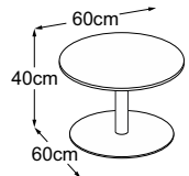
Center Leg 40 (Tischplatte: Struttur Grigio Antracite) Bestell-Nummer: DCL4SA4
