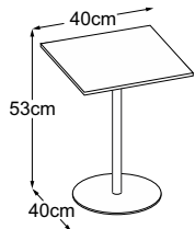
Center Leg 53 (Tischplatte: Vetro Bianco) Bestell-Nummer: DCL5VB6
