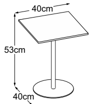
Center Leg 53 (Tischplatte: Struktura Grigio Antracite) Bestell-Nummer: DCL5SA6
