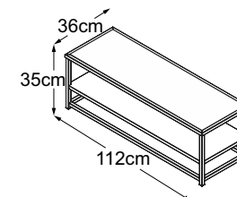
Lowboard (Piano del tavolo: Struttura Verde) Codice: DLOW1SV
