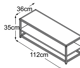
Lowboard (Piano del tavolo: Struttura Grigio Chiaro) Codice: DLOW1SC
