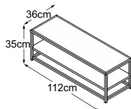
Lowboard (Piano del tavolo: Vetro Marrone) Codice: DLOW1VM
