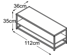
Lowboard (Tischplatte: Vetro Nero ) Bestell-Nummer: DLOW1VN
