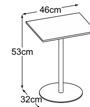
Center Leg 53 (Tischplatte: Struttura Grigio Chiaro) Bestell-Nummer: DCL5SC7
