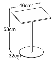
Center Leg 53 (Tischplatte: Struttura Grigio Antracite) Bestell-Nummer: DCL5SA7
