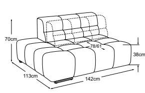
Penisola grande bracciolo dx incl. 1 SRM
