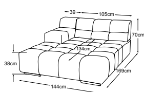
Penisola bracciolo sx
