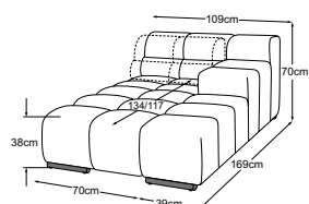
Penisola piccola bracciolo dx incl. 1 SRM
