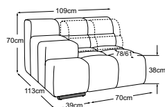
Elemento 70 bracciolo sx incl. 1 SRM
