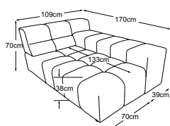
Longchair bracciolo dx
