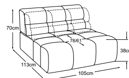
Elemento 105 senza bracciolo incl. 1 SRM
