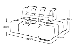
Elemento 2p con terminale dx incl. 1 SRM
