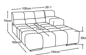
Penisola bracciolo dx
