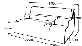
Élément 105 accoudoir droit incl. RMD
