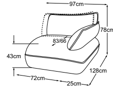
Element 70 armrest right incl. MBA Item number: D134120
