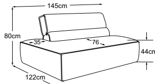
Elemento 2p con terminale sx Codice: D009520
