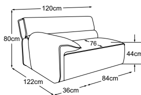
Elemento 105 bracciolo sx Codice: D009105
