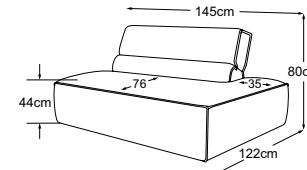
2HT rechts Bestell-Nummer: D009521
