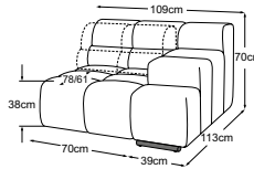
Element 70 armrest right incl.1 MBA
