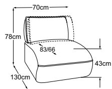
Element 70 ohne Armteil inkl. RVM Bestell-Nummer: D134118
