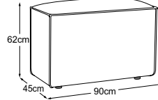
Back 90 Item number: D107902
