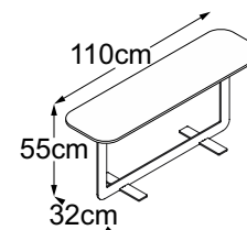
One Blade (Table top: Struttura Grigio Chiaro) Item number: D1L5SC8
