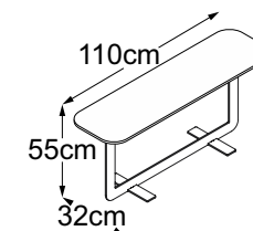
One Blade (Table top: Struttura Verde) Item number: D1L5SV8
