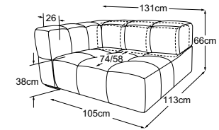
Element 105 armrest left incl. MBA Item number: D088123
