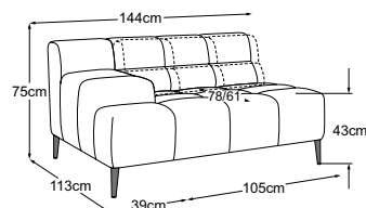
Elemento 105 bracciolo sx incl. SRM
