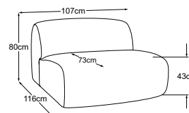
Elemento 105 senza bracciolo Codice: D074121
