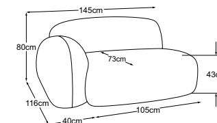
Elemento 105 bracciolo sx Bestell-Nummer: D074122
