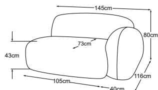
Elemento 105 bracciolo dx Codice: D074123
