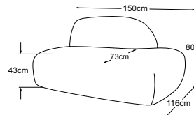
Elemento 2p con terminale dx Codice: D074521
