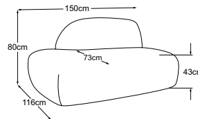
2HT links Bestell-Nummer: D074520
