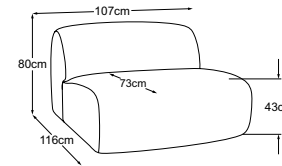
Element 105 ohne Armteil Bestell-Nummer: D074121
