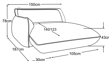
REC armrest left incl. MBA
