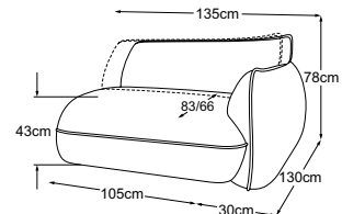
Element 105 armrest right incl. MBA
