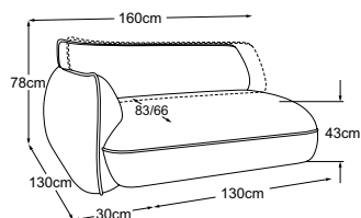
Elemento 130 bracciolo sx incl. 1 SRM Codice: D073126
