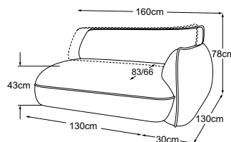
Elemento 130 bracciolo dx incl. 1 SRM Codice: D073127
