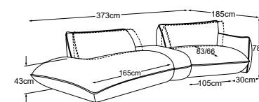
Elem. 2p con terminale sx + elemento trapezoidale + elemento 105 bracc. dx incl. 2 SRM Codice: D073661
