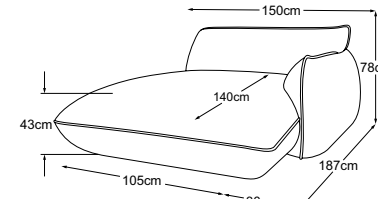
Penisola bracciolo dx Codice: D073131
