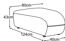
Elemento trapezoidale Codice: D073523
