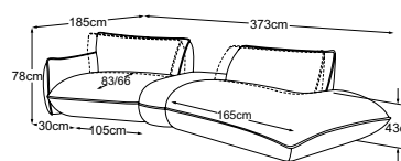
Elem. 105 bracc. sx + elemento trapezoidale + elemento 2p con terminale dx incl. 2 SRM Codice: D073660
