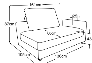
Elemento 140 bracciolo dx Codice: D071127
