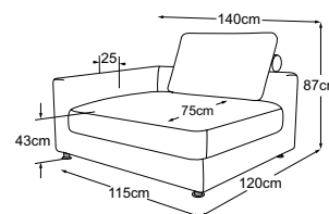
Elemento 120 profondo bracciolo sx Codice: D071101
