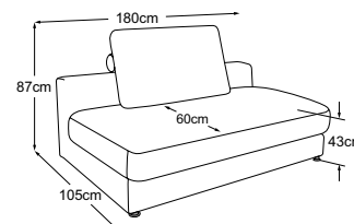
Elemento 180 Codice: D071117
