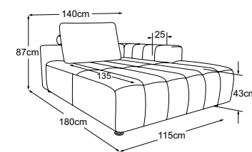
Penisola PS bracciolo dx* Codice: D071663*
