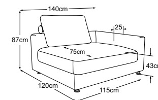
Elemento 120 profondo bracciolo dx Codice: D071102
