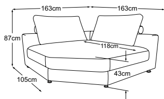
Angolo trapezoidale 105-120 Codice: D071522
