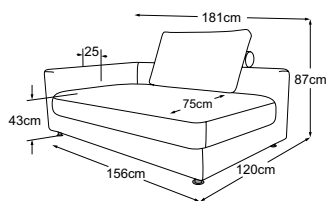
Elemento 160 profondo bracciolo sx Codice: D071129
