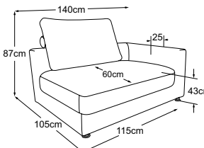
Elemento 120 bracciolo dx Codice: D071122
