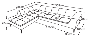
OTM-3 ohne Kissen Bestell-Nummer: D010563
